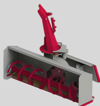
Снегомет шнеко- роторный
